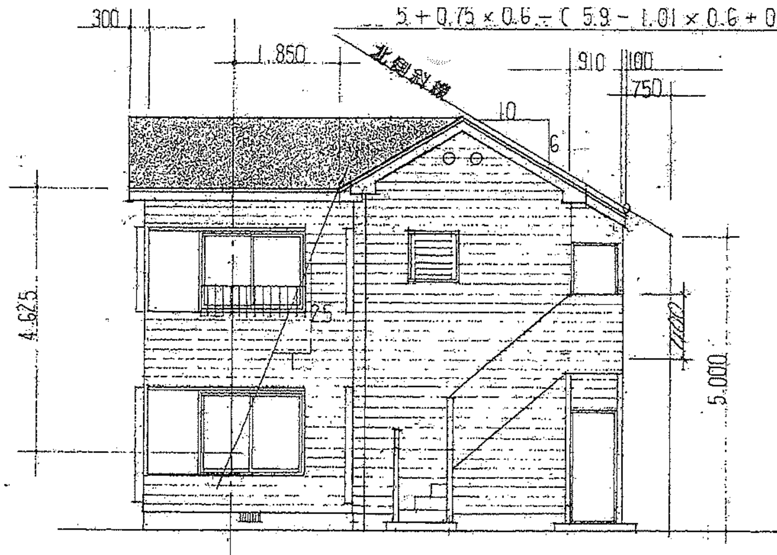
東立面図
