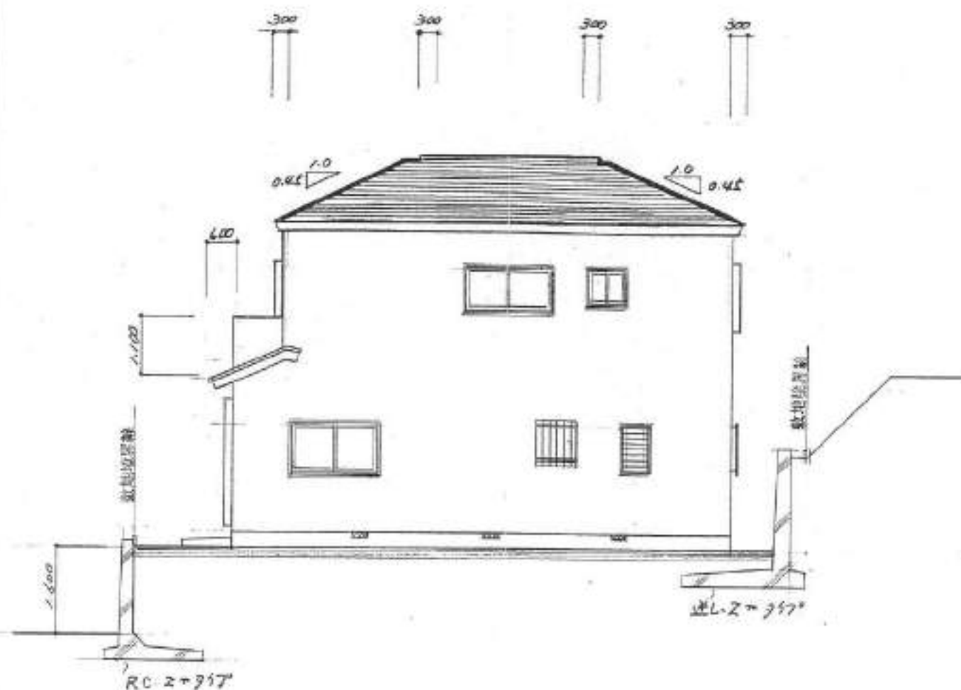
東立面図 S=1:100
