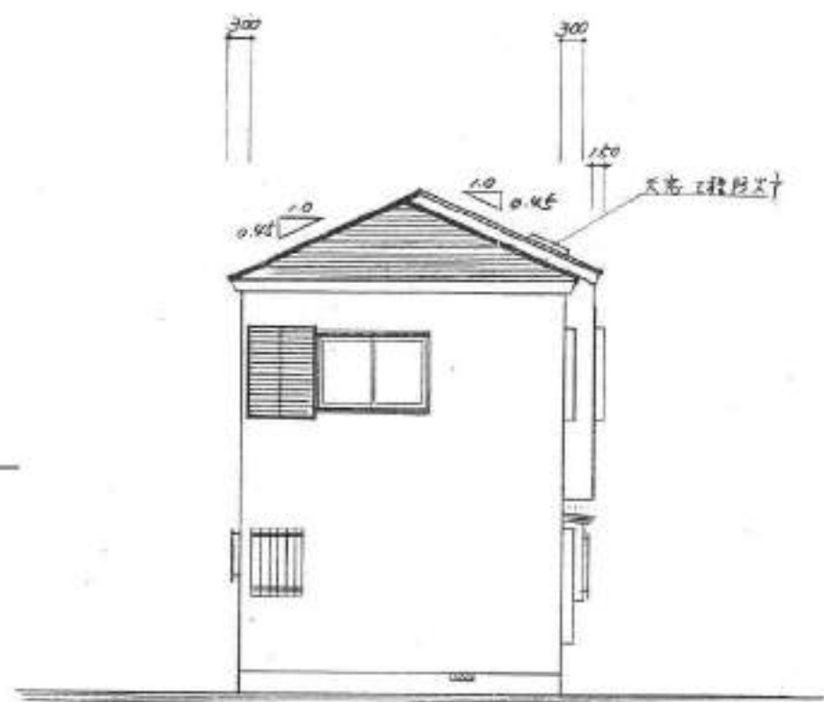
北立面図 S=1:100
